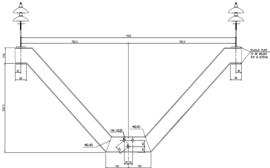
ELEVATION
